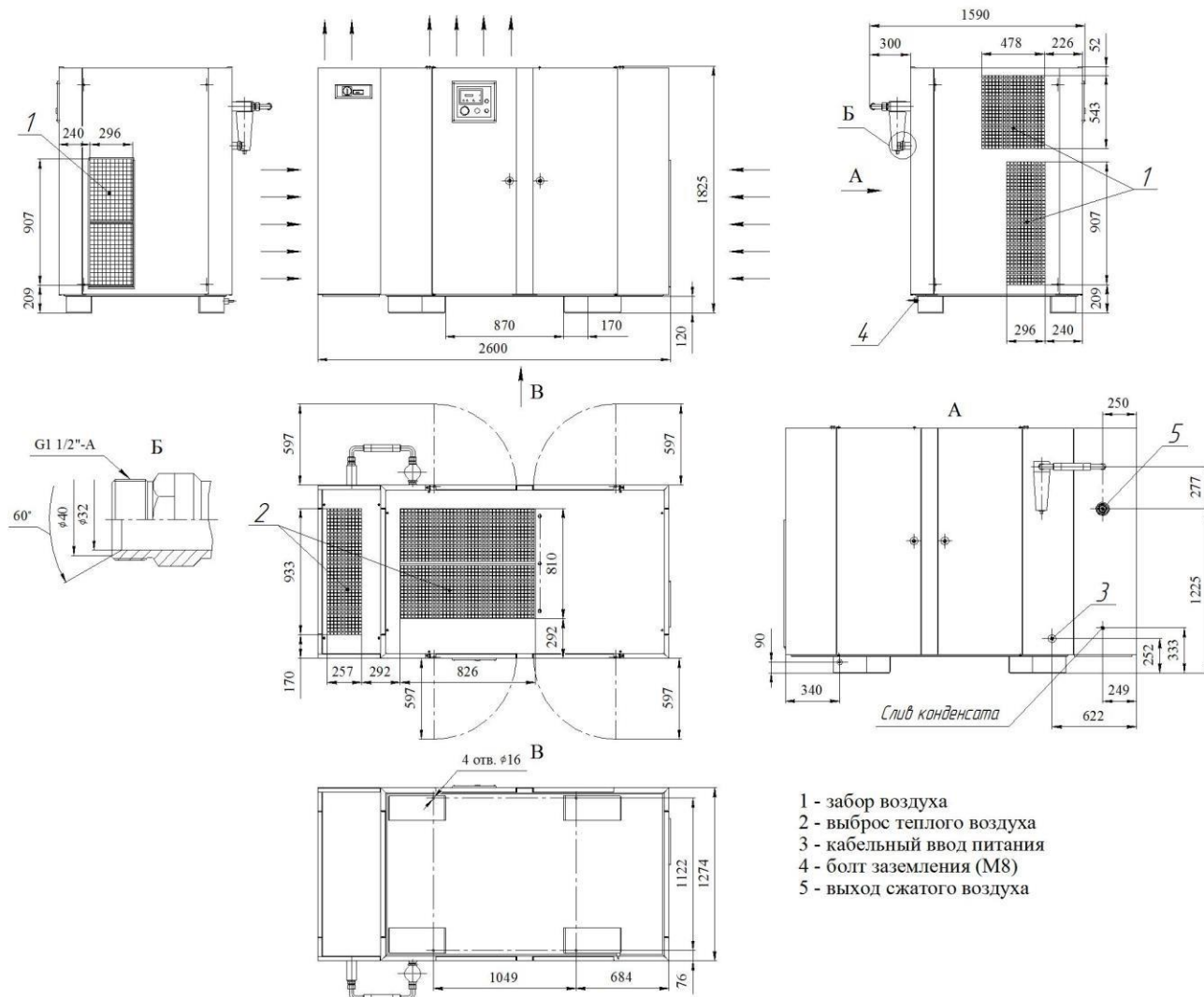
Установка компрессорная ВК60Р-ДВС. Установочные и присоединительные размеры.
