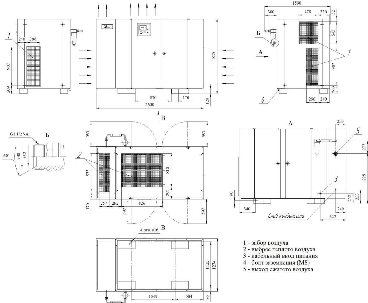
Установка компрессорная ВК60P-Д. Установочные и присоединительные размеры.
